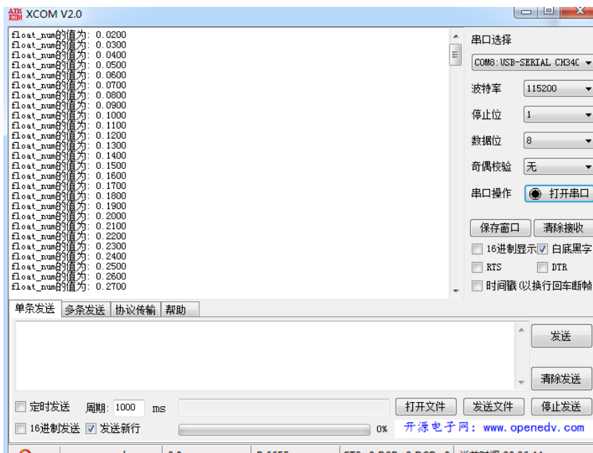
图 1.4.1 串口输出
