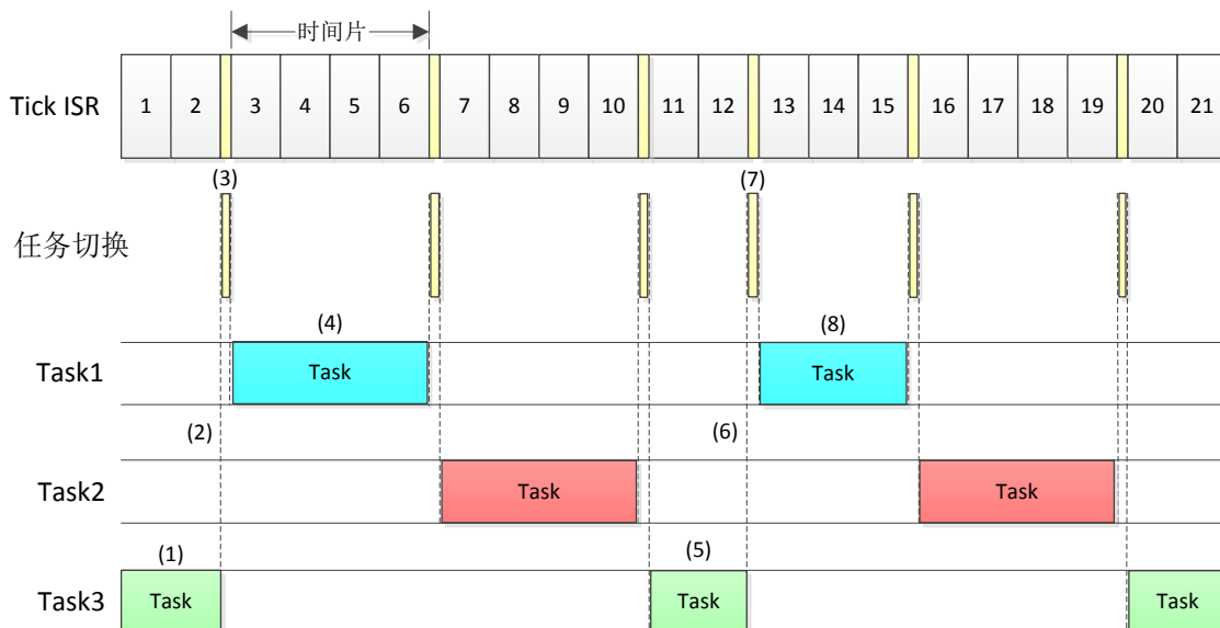
图 5.6.1 轮转调度
