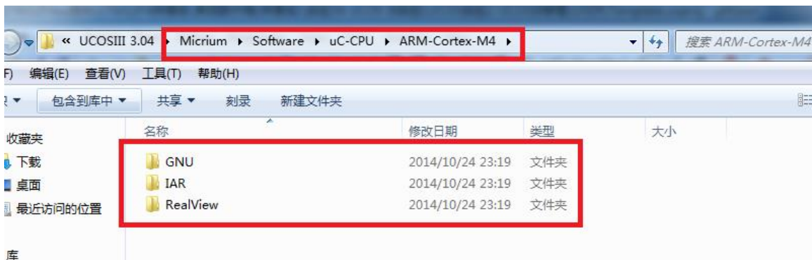
图 4.2.6 ARM-Cortex-M4 文件夹
